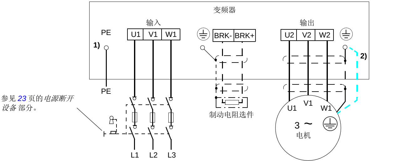
接线图
