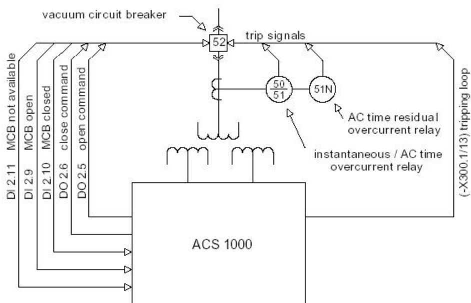
图10-2 真空断路器的主接线图
