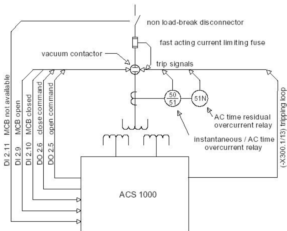
图10-3 真空控制器的主接线图
