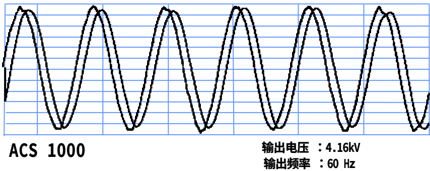
图 3-2 变频器输出电压和电流波形图
