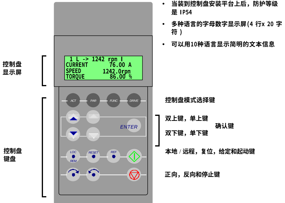
图 3-8 CDP 312 控制盘
