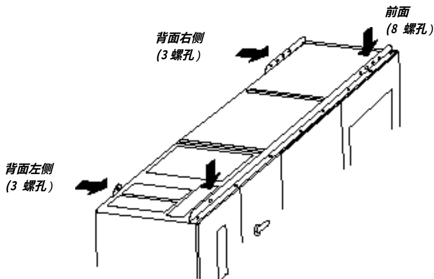
图10-7 安装起重轨
