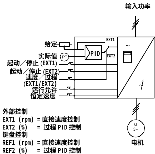
控制图 图 4-7 PID控制宏的控制图
