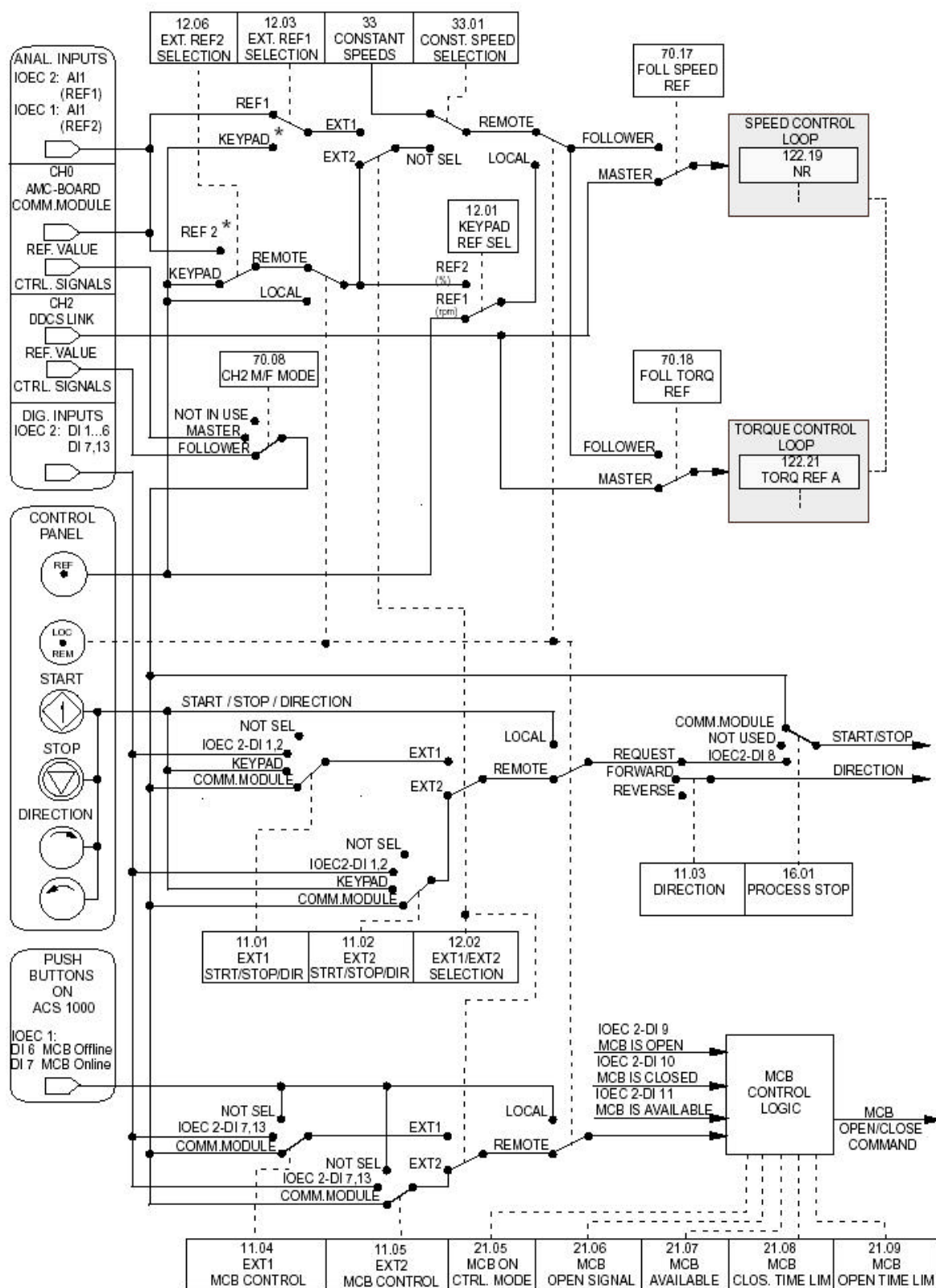
图4-15 从机控制信号图
