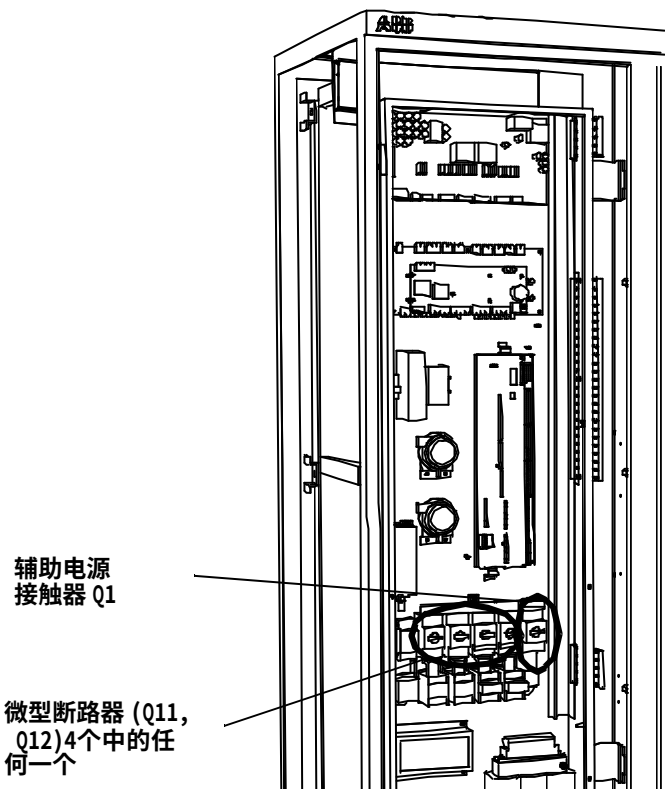
图 7-1 控制柜
