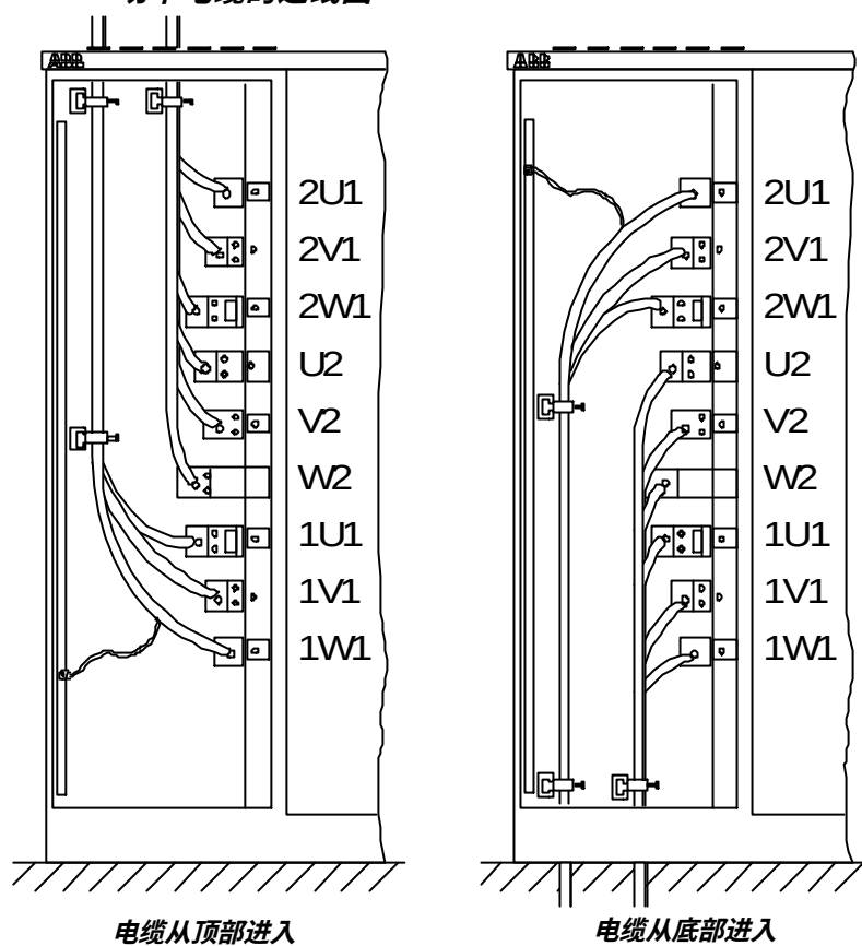
图 10-12 功率电缆的进线图
