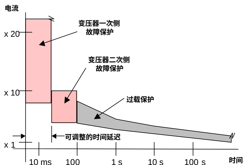
图 10-4 保护设计图
