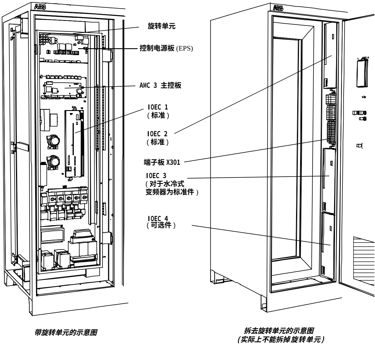
图 4-2 IOEC板的定位
