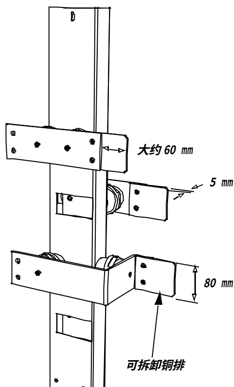
图10-17 带可拆卸铜排的功率端子
